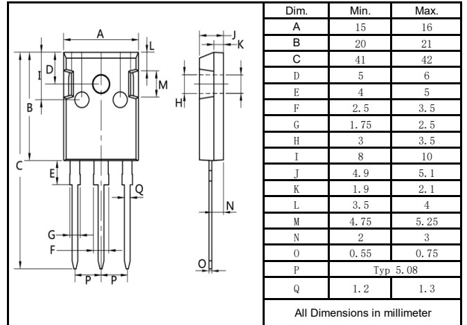
T0-247
